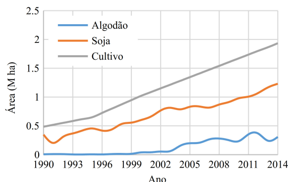
Figura 2. Evolução da área plantada total (soma das áreas nas bacia Rio Grande, Carinhanha e Correntes) de soja, algodão e cultivo.
