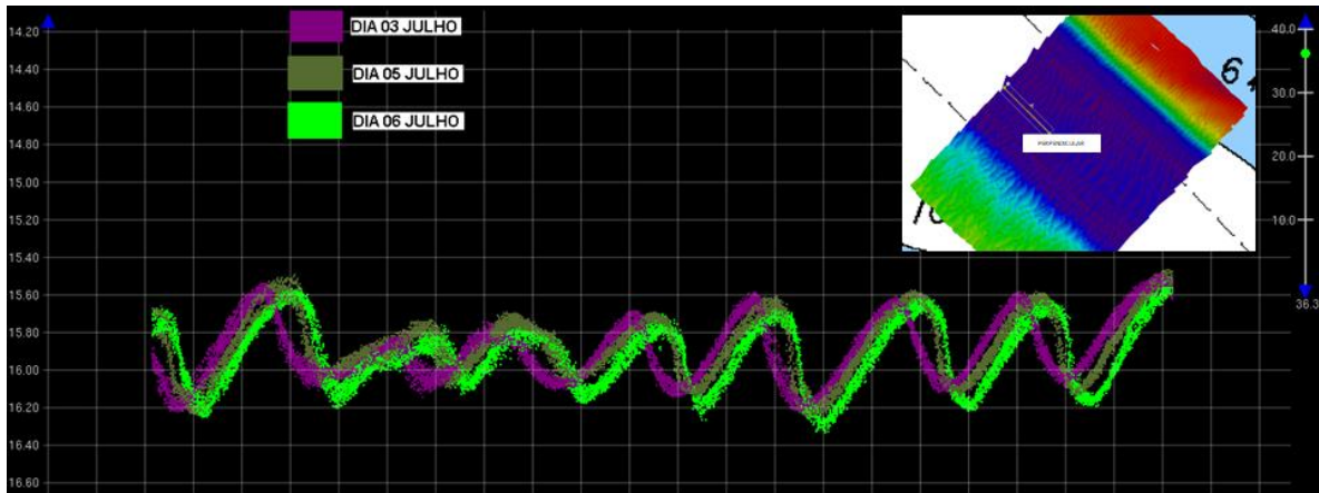
Figura 1. Corte vertical perpendicular à direção do feixe de varredura e portanto perpendicular ao deslocamento das ondas de areia. Cada um dos dias, representados em cor diferente, apresenta uma superfície coerente. Considerados em conjunto o deslocamento das feições tende a misturar a variancia do fenômeno na janela de tempo com a incerteza vertical da medição.
