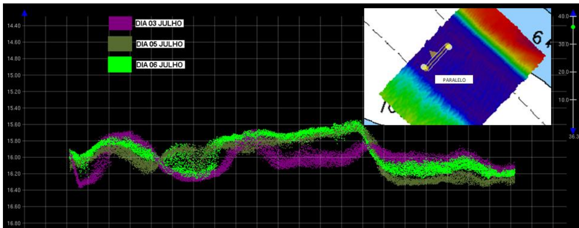
Figura 2. Corte vertical paralelo à direção do feixe de varredura. Os perfis relativos a cada dia isolado, representados cada qual com sua cor, não conseguem exprimir a morfologia do piso submerso, assim como seu conjunto inibe a ideia de deslocamento.
