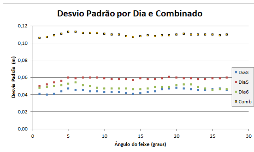
Figura 3. Gráfico do desvio padrão por ângulo de abertura do feixe, para cada dia de levantamento e para a superfície combinada dos três dias.
