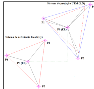
Fig 1 – Transformação de local (x, y) para UTM (E, N)
