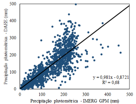
Fig. 2 - Relação entre os dados de precipitação observada e estimada por meio do produto GPM_3IMERGM v04, para o ano de 2015.
