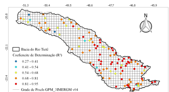
Fig. 3 - Valores de R^2 para cada pluviômetro no interior da Bacia do Rio Tietê.
