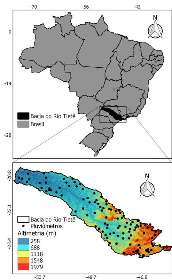
Fig. 1 - Localização da Bacia do Rio Tietê e distribuição dos pluviômetros no interior da bacia.
