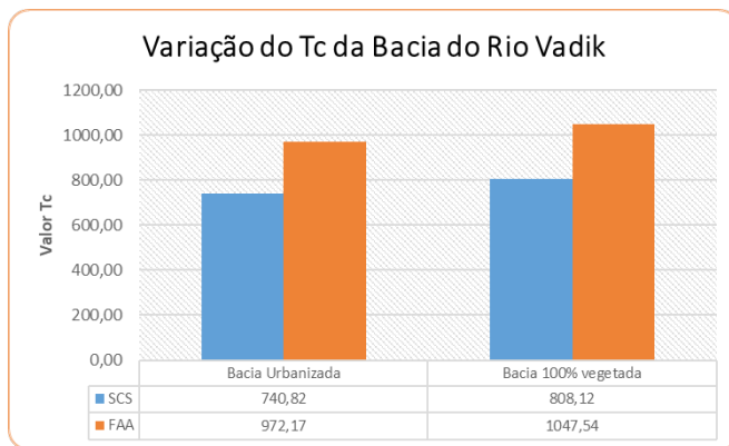
Fig. 3- Variação do Tc na área de estudos
