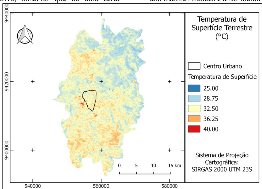
Figura 3 - Temperatura de Superfície Terrestre do município de Presidente Dutra-MA
