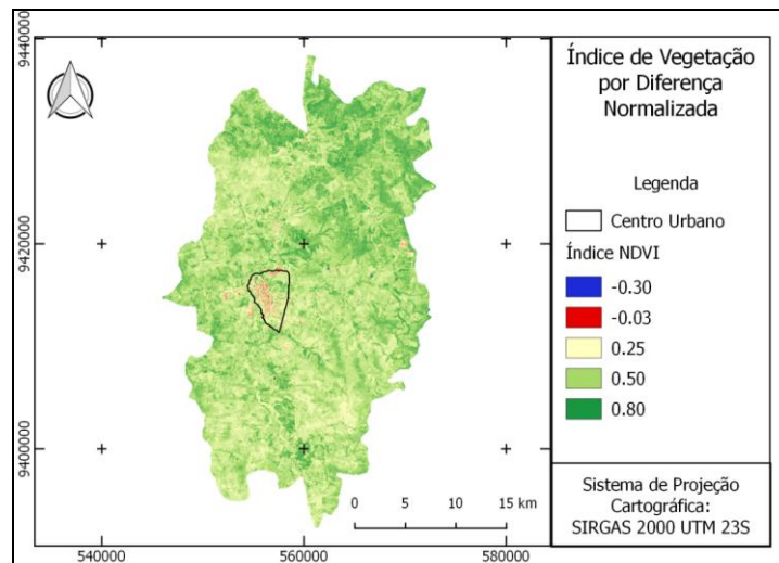
Figura 2 – Índice de Vegetação por diferença Normalizada do município de Presidente Dutra-MA
